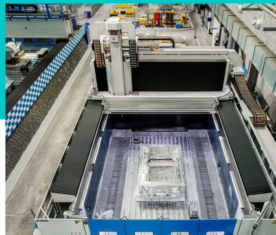
3 000 m 2 d'ateliers climatisés au degré près, dotés de plusieurs tours verticaux et aléseuses, de 3 centres d'usinage grande vitesse et d'une fraiseuse double portique pouvant usiner des pièces jusqu'à 10 m de large et 30 m de long.
